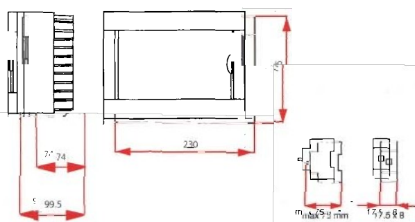
Внешний бокс на 8 автоматов 90912108
